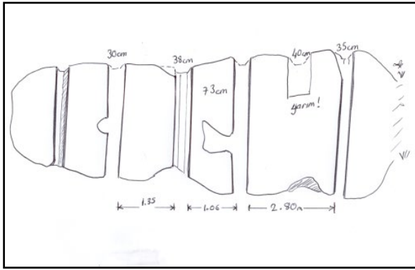
Plan/Kesit-Çizim 1: Dumanlı Dağı orman örtüsü içerisinde bulunan sunak kayalıkları.
